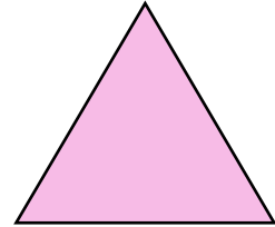
LIKSIDIG TRIANGEL Alla sidor är lika långa
