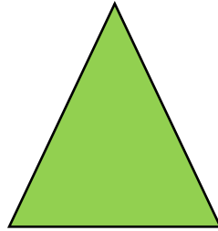
LIKBEIT TRIANGEL Två av sidorna är lika långa
