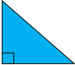
RÄTVINKLIG TRIANGEL En av vinklarna är rät ( 90^\circ )
